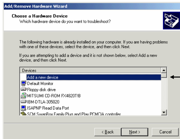
Bild 5.2-3: Auswahl für Einrichten neuer Hardware
